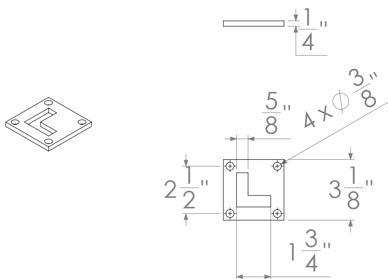
Flange
