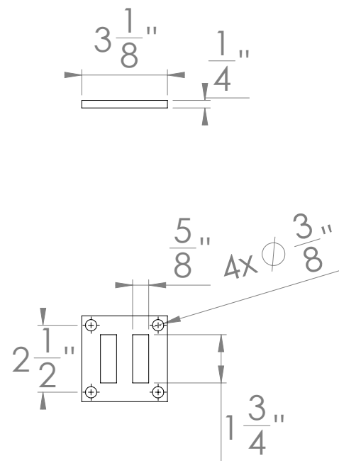
Flange
